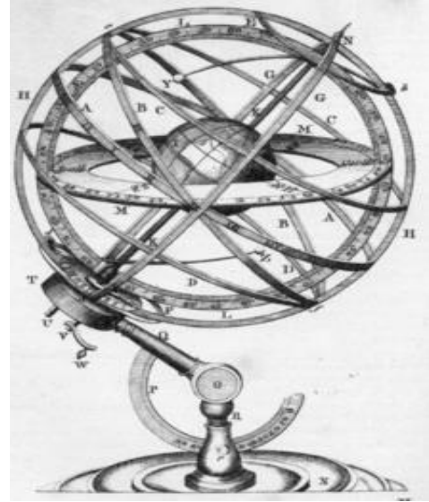
Hipparchus'un Kullandığı Çemberli Küre Diyagramı
